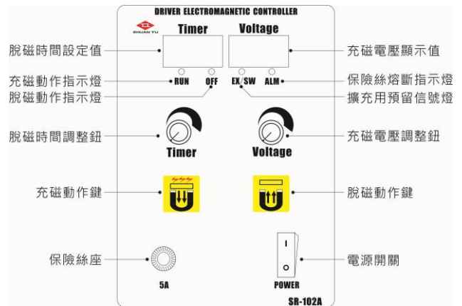
按鍵開關型
